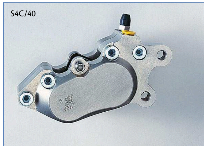
4-Kolbenzange, Classic, silber, hartcoatiert. Mit TÜV. 4-piston caliper, Classic, silver, hard-anodized. With TÜV.
