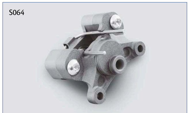
S064 2-Kolbenzange hinten mit Aufnahme 64 mm. 2-piston calliper rear with 64 mm pattern.
