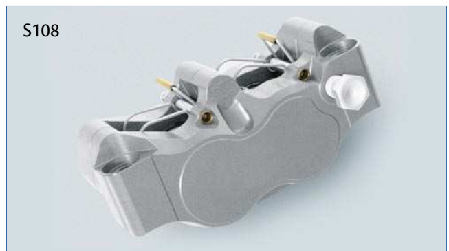
S108 4-Kolben-Zange mit Radial-Aufnahme 108 mm, 23 mm Versatz. Passend für alle Modelle mit BREMBO Racing Radial Bremszange. 4-piston calliper with 108 mm, 23 mm backfill radial pattern. Suitable for all models with BREMBO racing radial callipers.
